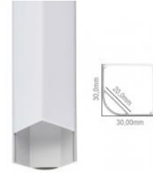
Perfil de Aluminio para Tira de LEDs - Difusor Opal - Tira de 2 Metros
